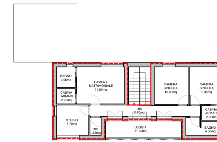
Pianta piano primo (+3.10m)
